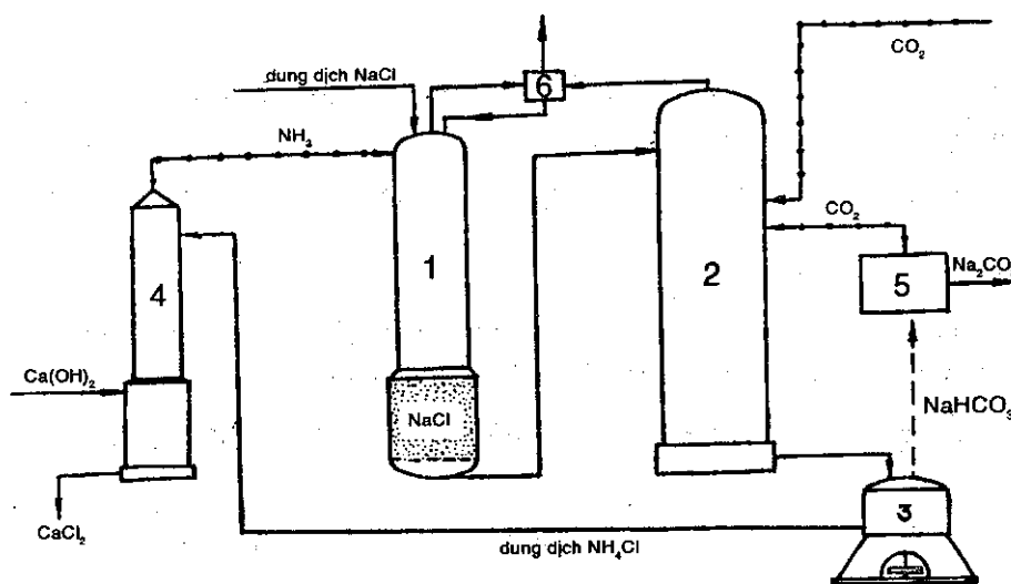
Sơ đồ 2.7. Nguyên lí sản xuất natri bicarbonat theo phương pháp Solvay
