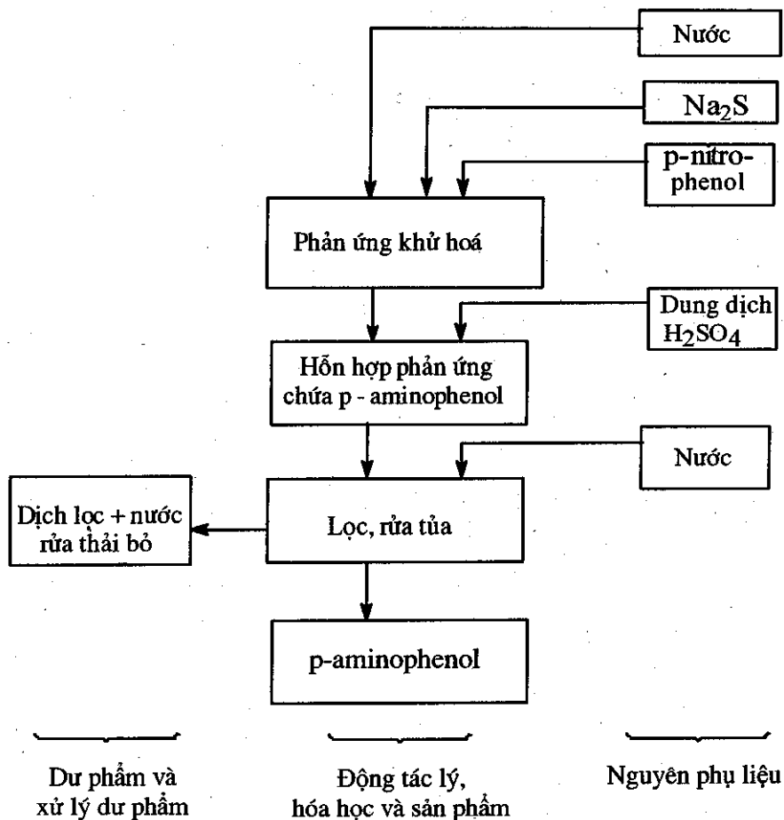
Sơ đồ 1.2. Qui trình sản xuất p-aminophenol từ p-nitrophenol.
