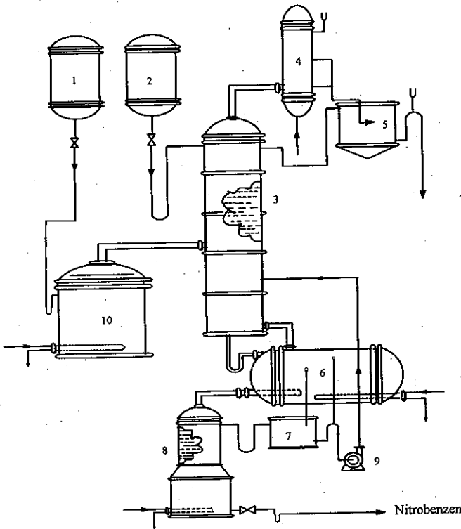
Sơ đồ 1.5. thiết bị điều chế nitrobenzen theo phương pháp liên tục
