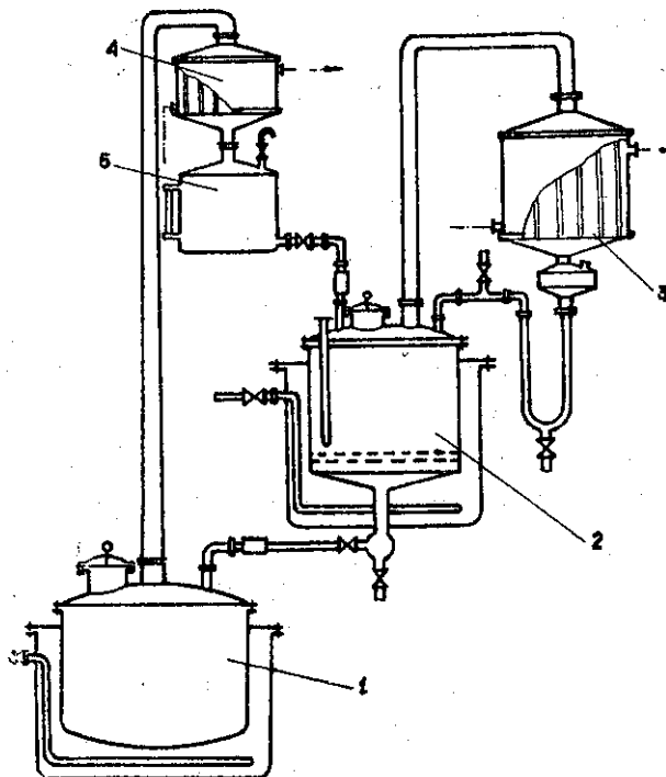
Sơ đồ 2.6. Thiết bị chiết lecithin 1. Nồi cất cách thủy; 2. Bình chiết; 3, 4. Sinh hàn; 5. Bình chứa cồn.
