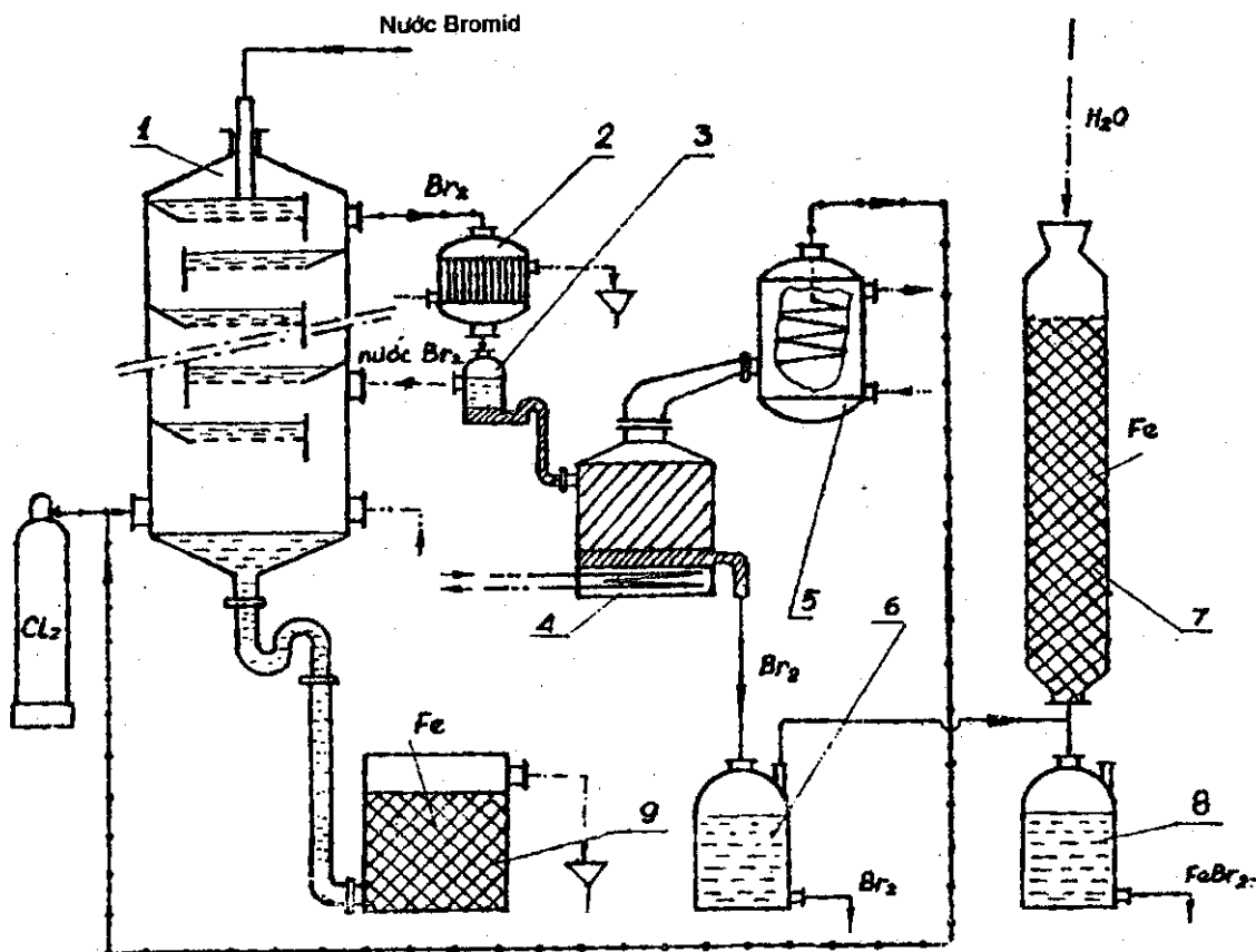
Sơ đồ 2.2. Thiết bị sản xuất Brom
