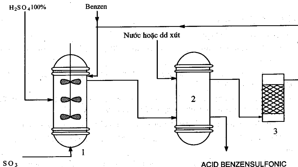
Sơ đồ 1.6. Thiết bị điều chế acid benzensulfonic theo phương pháp liên tục
