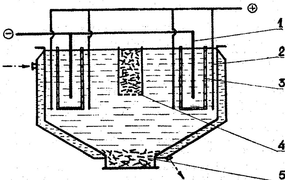
Sơ đồ 2.5. Cấu tạo bình điện phân sản xuất KMnO 4
