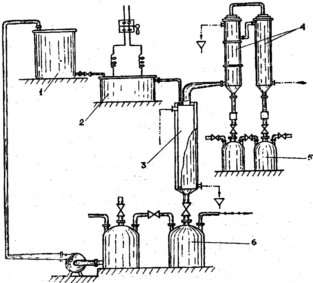
Sơ đồ 2.4. Thiết bị sản xuất \text{H}_2\text{O}_2 bằng phương pháp điện hoá
