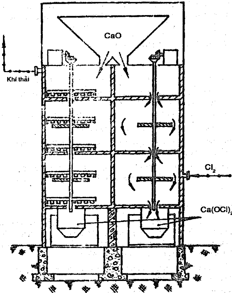
Sơ đồ 2.3. Thiết bị sản xuất Ca(ClO) 2
