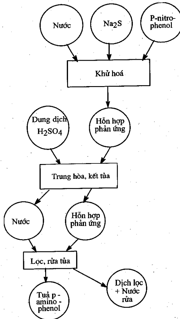
Sơ đồ 1.3. Quy trình sản xuất p-aminophenol từ p-nitrophenol
