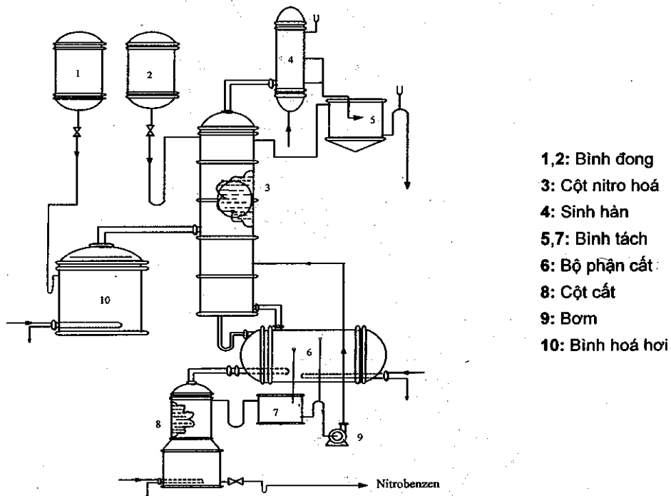
Sơ đồ 1.4. Thiết bị điều chế nitrobenzen theo phương pháp liên tục
