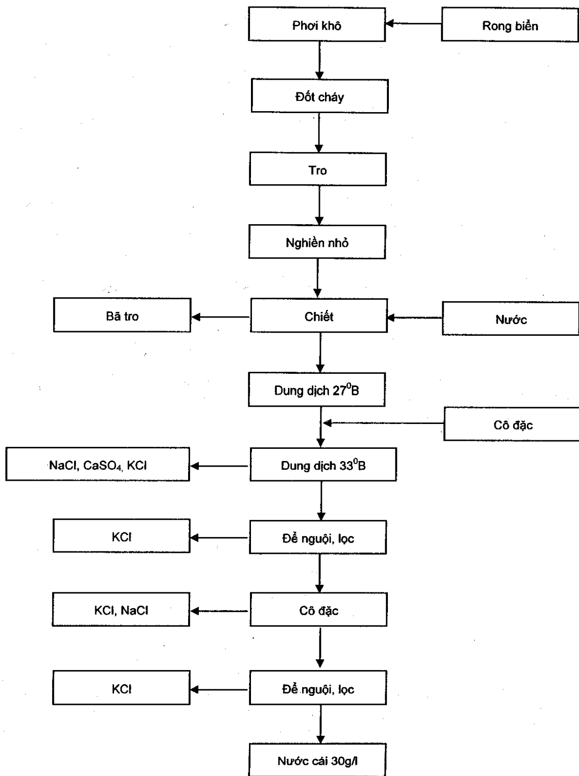
Sơ đồ 2.1. Quy trình tạo dung dịch đậm đặc iod hoà tan
