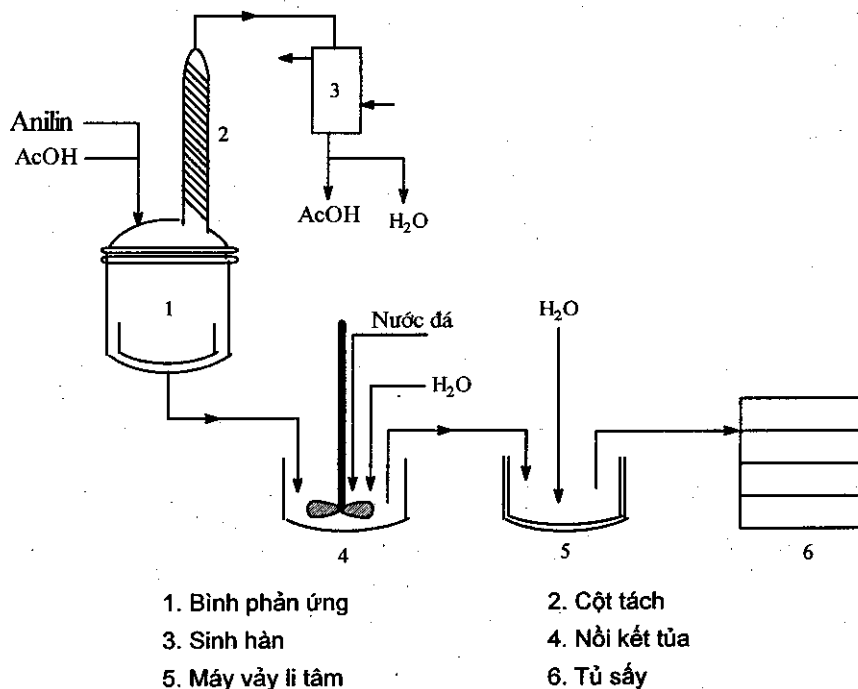
Sơ đồ 1.7. Thiết bị điều chế acetanilid
