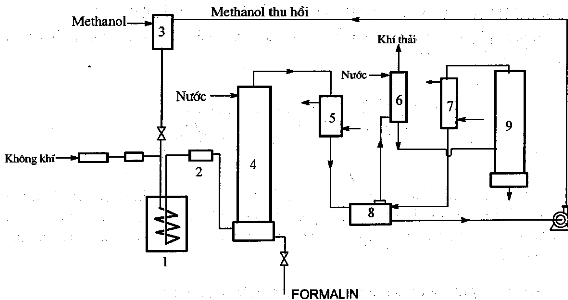
Sơ đồ 1.8. Nguyên lí thiết bị phản ứng điều chế formandehyd từ methanol
