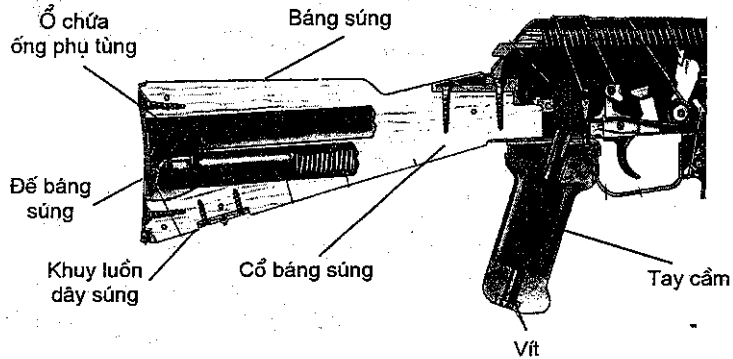
Hình 3.13. Báng súng và tay cầm
