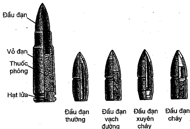
Hình 3.17. Đạn súng tiểu liên (K56)
