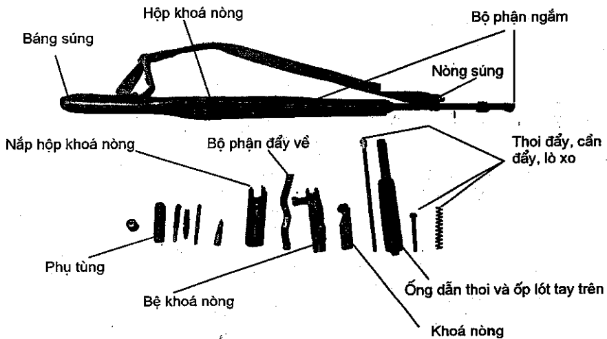
Hình 3.30. Cấu tạo của súng trường CKC
