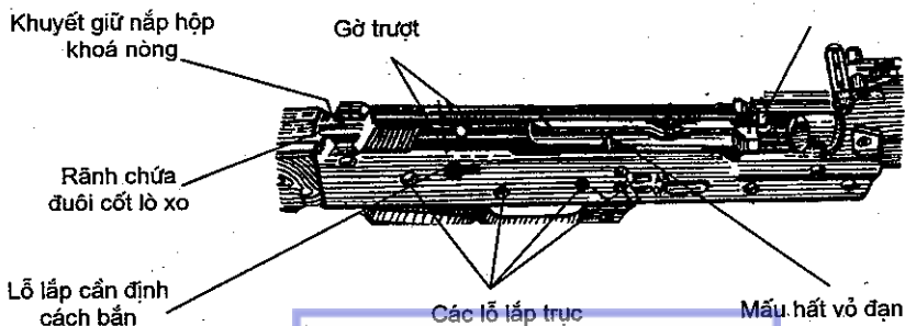
Hình 3.6. Hộp khoá nòng
