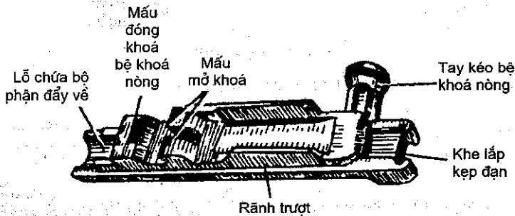
Hình 3.35. Bộ khoá nòng
