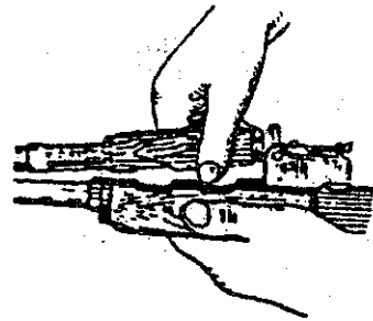
Hình 3.23. Tháo ống dẫn thoi và ốp lót tay trên
