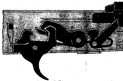
Hình 3.26. Vị trí các chi tiết của bộ phận cò khi lên đạn, khoá an toàn ở vị trí bắn
