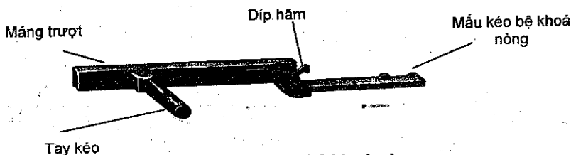
Hình 3.58. Tay kéo bệ khoá nòng
