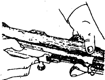
Hình 3.46. Tháo bộ phận đẩy về
