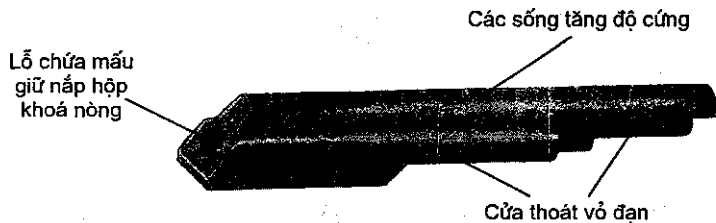
Hình 3.7. Nắp hộp khoá nòng
