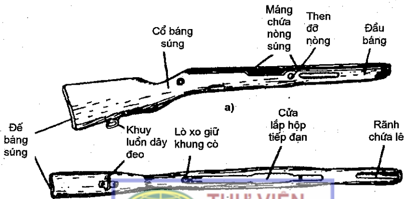
Hình 3.41. Báng súng
