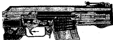
Hình 3.27. Vị trí các bộ phận cò khi bắn
