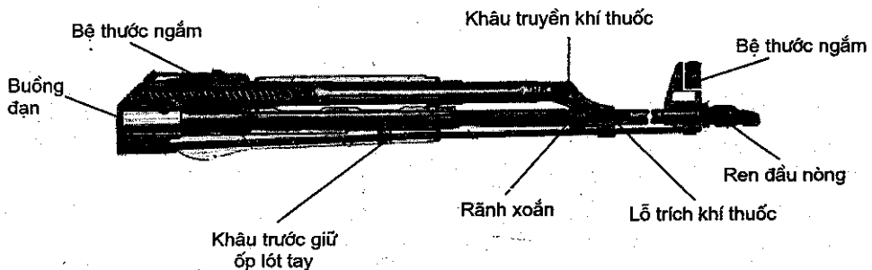
Hình 3.2. Nòng súng
