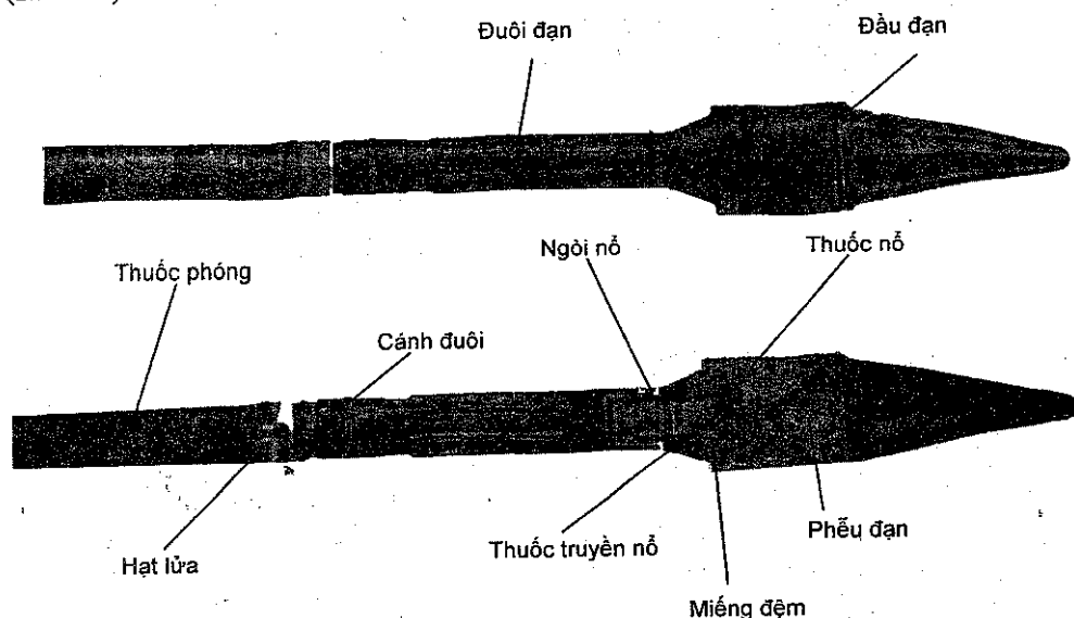
Hình 3.69. Đạn B40 TRƯỜNG ĐẠI HỌC HUBT TÀI LIỆU PHỤC VỤ THAM KHẢO NỘI BỘ
