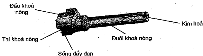
Hình 3.9. Khoá nòng
