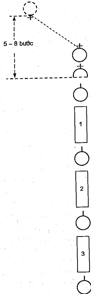
Hình 1.14. Đội hình trung đội một hàng dọc
