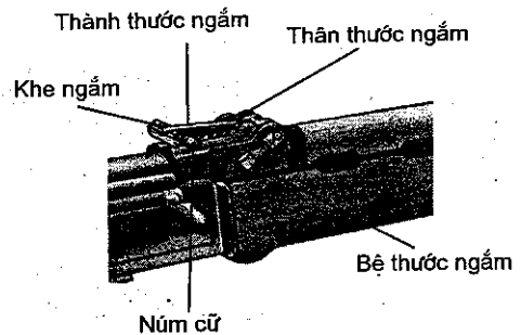
Hình 3.5. Thước ngắm
