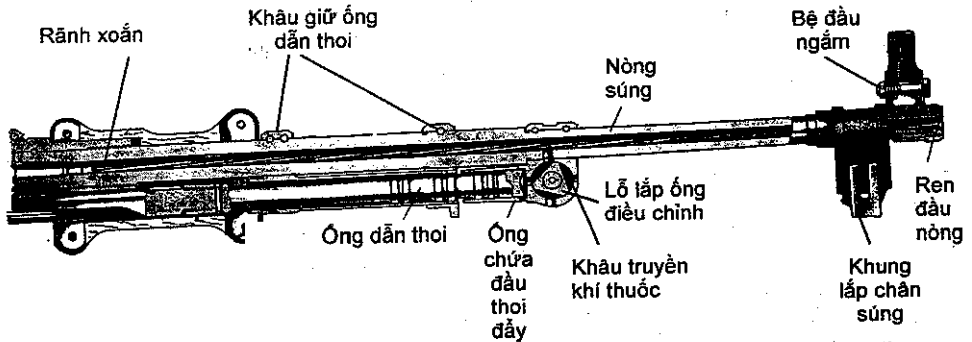
Hình 3.52. Nòng súng
