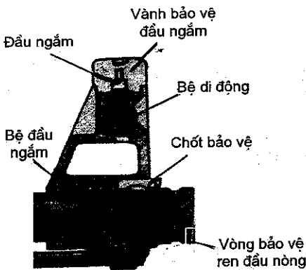
Hình 3.4. Đầu ngắm
