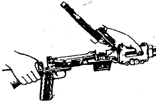
Hình 3.66. Tháo bộ phận cò và băng súng
