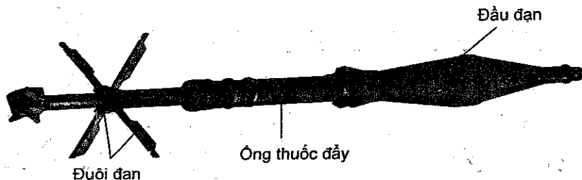
Hình 3.78. Đạn súng diệt tăng B41 THƯ VIỆN HUBT TÀI LIỆU PHỤC VỤ THAM KHẢO NỘI BỘ
