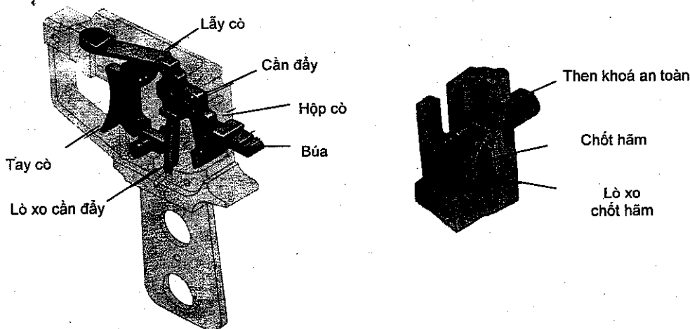
Hình 3.80. Bộ phận cò
