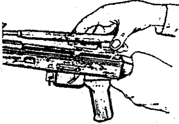
Hình 3.22a. Tháo bệ khoá nòng
