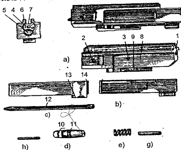
Hình 3.57. Khoá nòng
