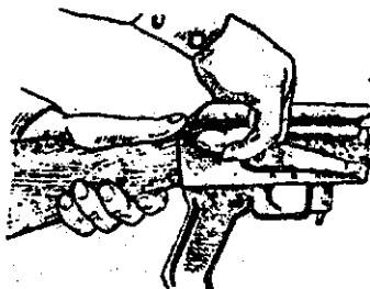
Hình 3.21a. Tháo nắp hộp khoá nòng
