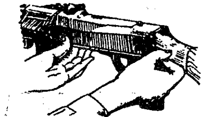
Hình 3.65. Tháo thông nòng
