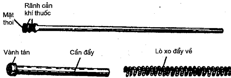
Hình 3.39. Thoi đẩy, cần đẩy và lò xo cần đẩy
