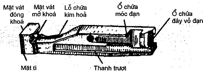
Hình 3.36. Khoá nòng
