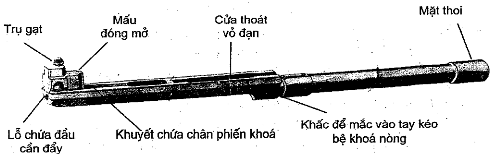
Hình 3.56. Bộ khoá nòng và thoi đẩy
