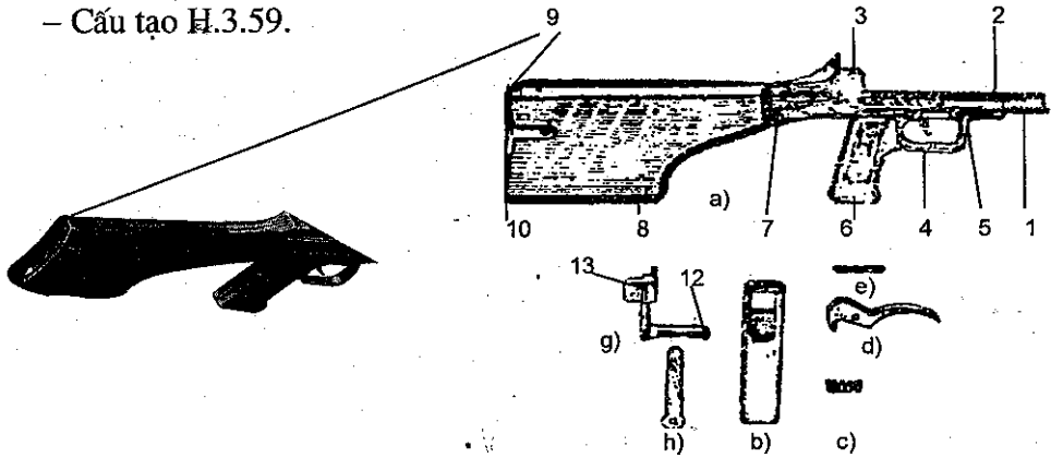
Hình 3.59. Bộ phận cò và báng súng
