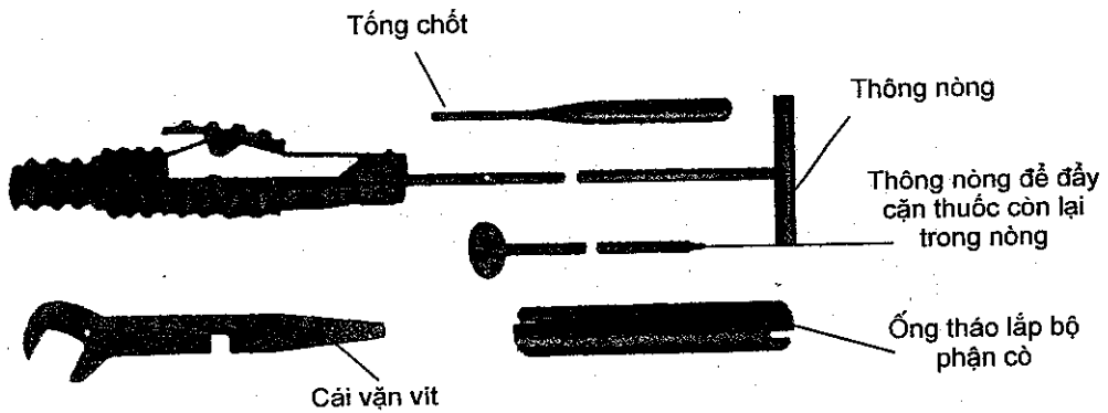
Hình 3.84. Phụ tùng
