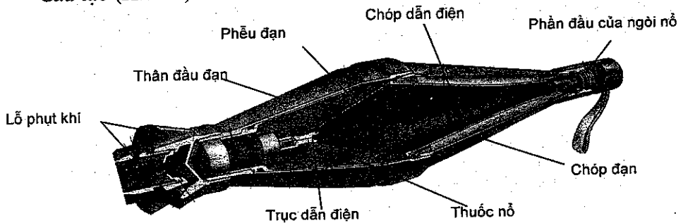
Hình 3.85. Đầu đạn
