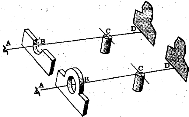
Hình 10.4. Đường ngắm đúng
