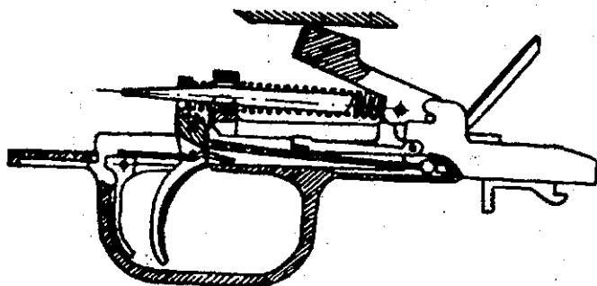
Hình 3.49. Vị trí các chi tiết bộ phận cơ khi khoá nòng lùi về sau
