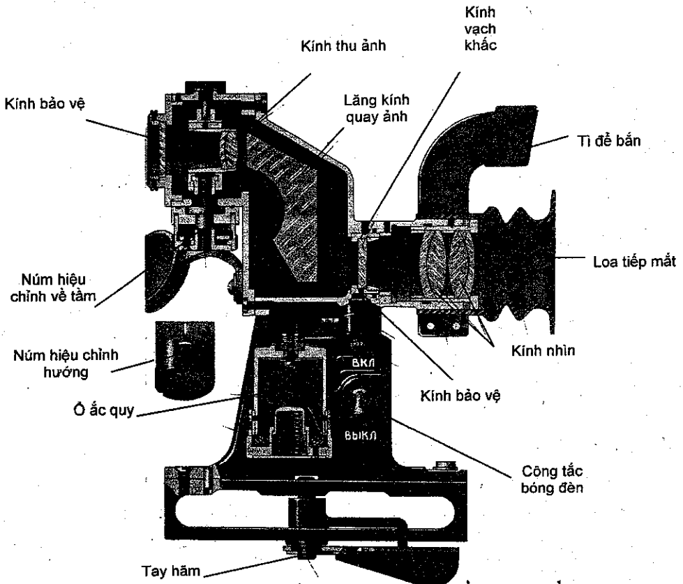
Hình 3.82. Kính ngắm quang học
