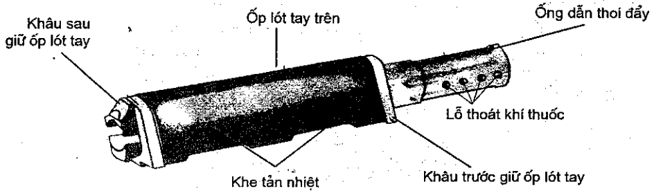
Hình 3.12. Ốp lót tay và ống dẫn thoi
