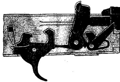
Hình 3.25. Vị trí các chi tiết của bộ phận cò trước khi lên đạn
