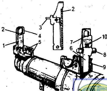
Hình 3.79. Bộ phận ngắm cơ khí 1. Thân đầu ngắm ; 2. Đầu ngắm dấu (-). Đầu ngắm dấu (+) ; 4. Vòng bảo vệ ; 5. Khung bảo vệ đầu ngắm khi gập ; 6. Thân thước ngắm ; 7. Khe ngắm ; 8. Cữ ngắm ; 9. Khung bảo vệ thước ngắm khi gập ; 10. Lỗ bầu dục.
