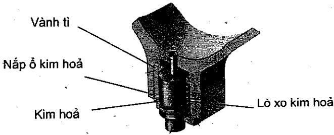
Hình 3.81. Bộ phận kim hoả
